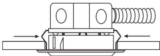
Рис. 2. Установка RMK400AP в подвесном потолке
